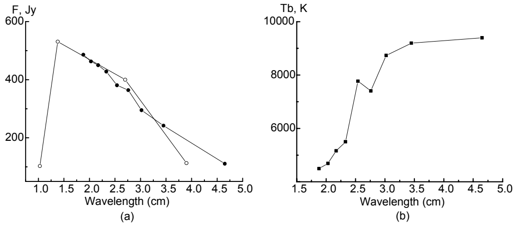
Рис. 6. (а) Спектры потоков F (Jy) радиоизлучения протуберанца по данным наблюдений на Южном (●) и Северо-восточном секторах (○) РАТАН-600; (б) спектр яркостных температур T_b по данным наблюдений на Южном секторе. (Каждая точка графика соответствует значению, полученному после осреднения данных по восьми соседним каналам радиометра).
