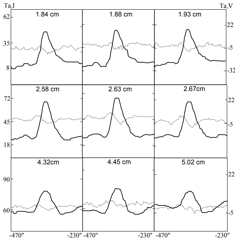
Рис. 7. Фрагменты записей интенсивности ( I , сплошные линии) и поляризации ( V , пунктирные линии) радиоизлучения протуберанца на ряде волн. По оси ординат на каждом рисунке отложены значения антенной температуры в градусах Кельвина, слева I , справа V .
